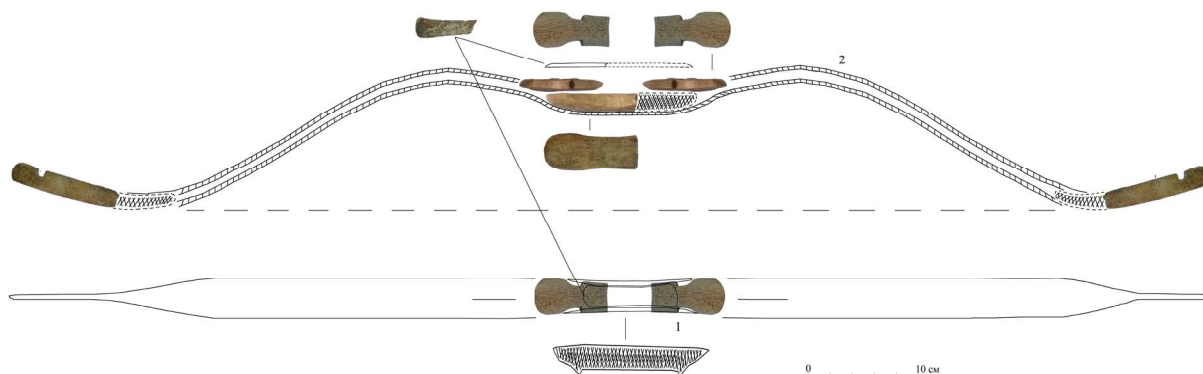
2-расм. Мураккаб таркибли камон конструкцияси. Рис. 2. Конструкция сложносоставного лука. Figure 2. Composite bow design.
